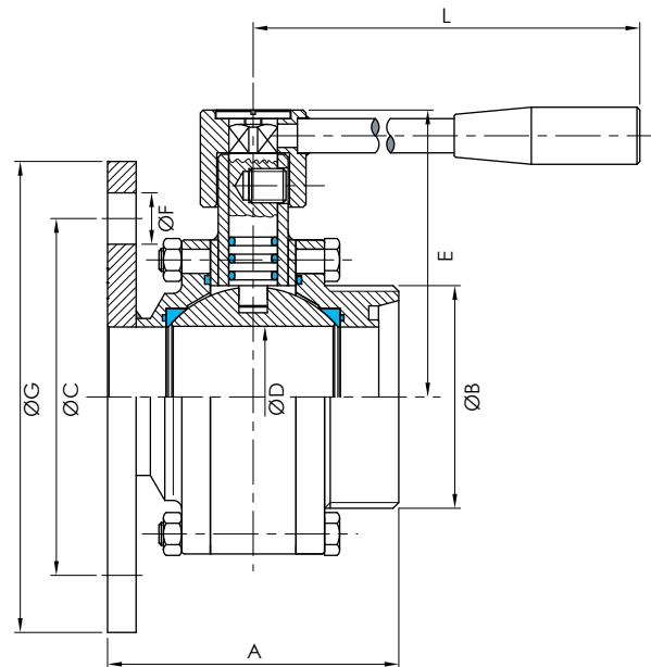
Posizione dei fori flangia rispetto alla valvola Position of the flange holes welded to the valve
